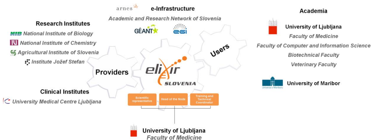
Slika 1: Struktura ELIXIR-SI
