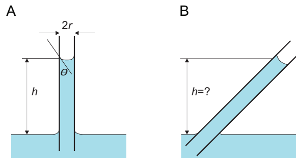
Slika 3.1: A) Shematski prikaz kapilarnega dviga v navpični kapilari. Višina kapilarnega dviga ( h ) je razlika med zunanjo gladino in gladino v kapilari. B) Kako visok je kapilarni dvig v nagnjeni kapilari?
